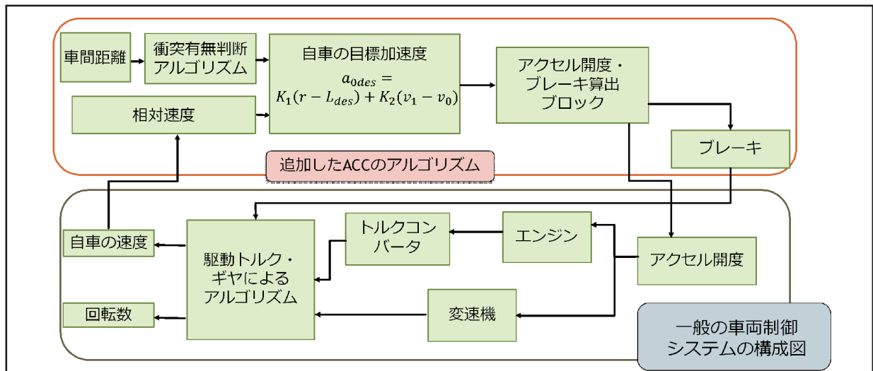
図4 ACCによる車両制御システム
