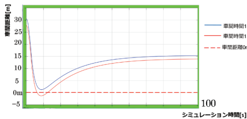
図9 速度 100km/h の車間距離の変動グラフ
