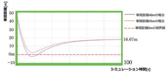
図10 車間距離 40m, 45m の場合の車間距離の変動グラフ
