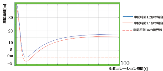
図8 速度 120km/h の車間距離の変動グラフ
