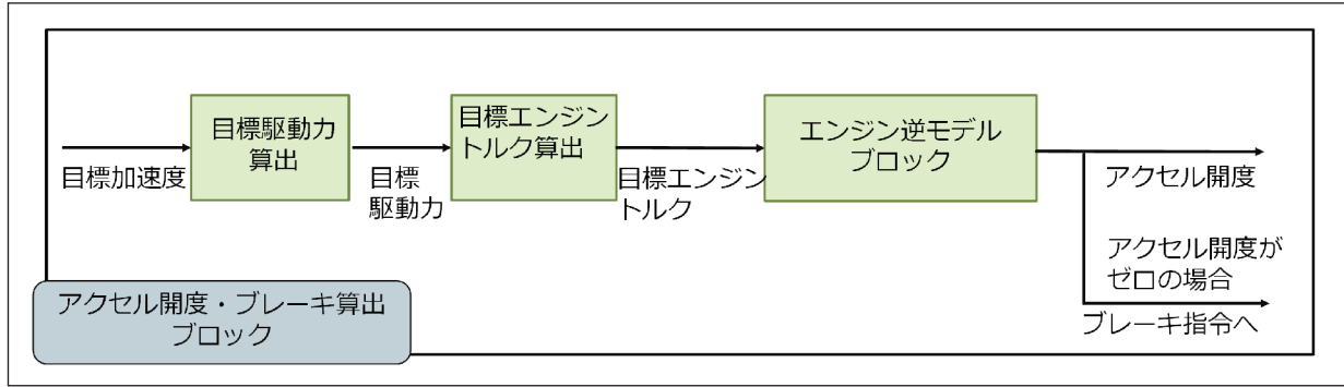
図5 アクセル開度・ブレーキ制御システム
