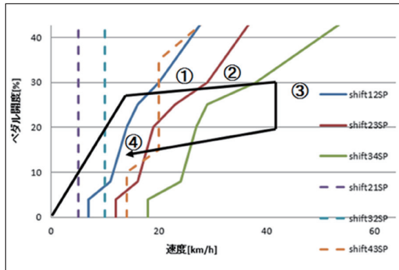
図3 変速制御のギヤ段シフト
