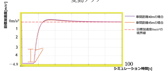
図11 車間距離 40m, 45m の場合の目標加速度の変動グラフ
